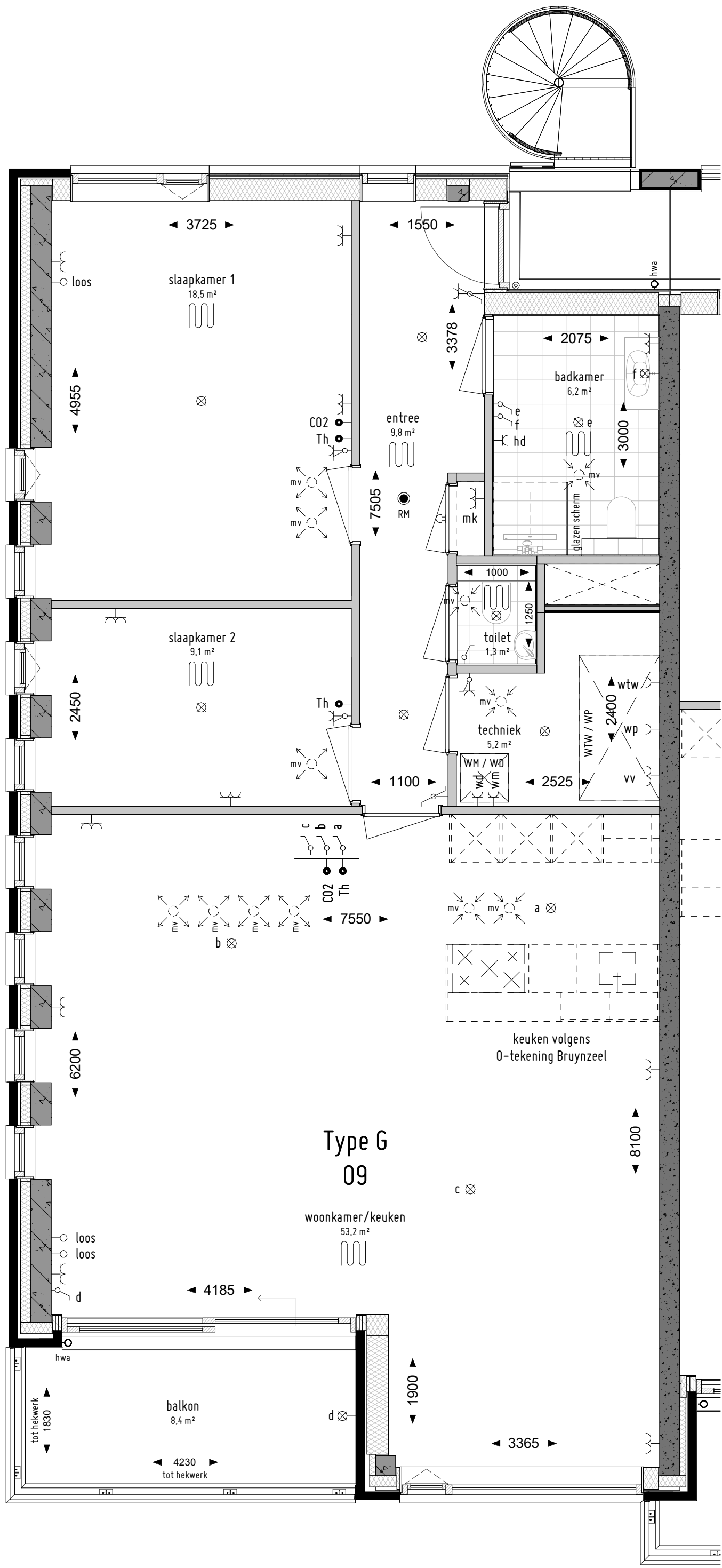
Bouwnummer 09 1 : 50
