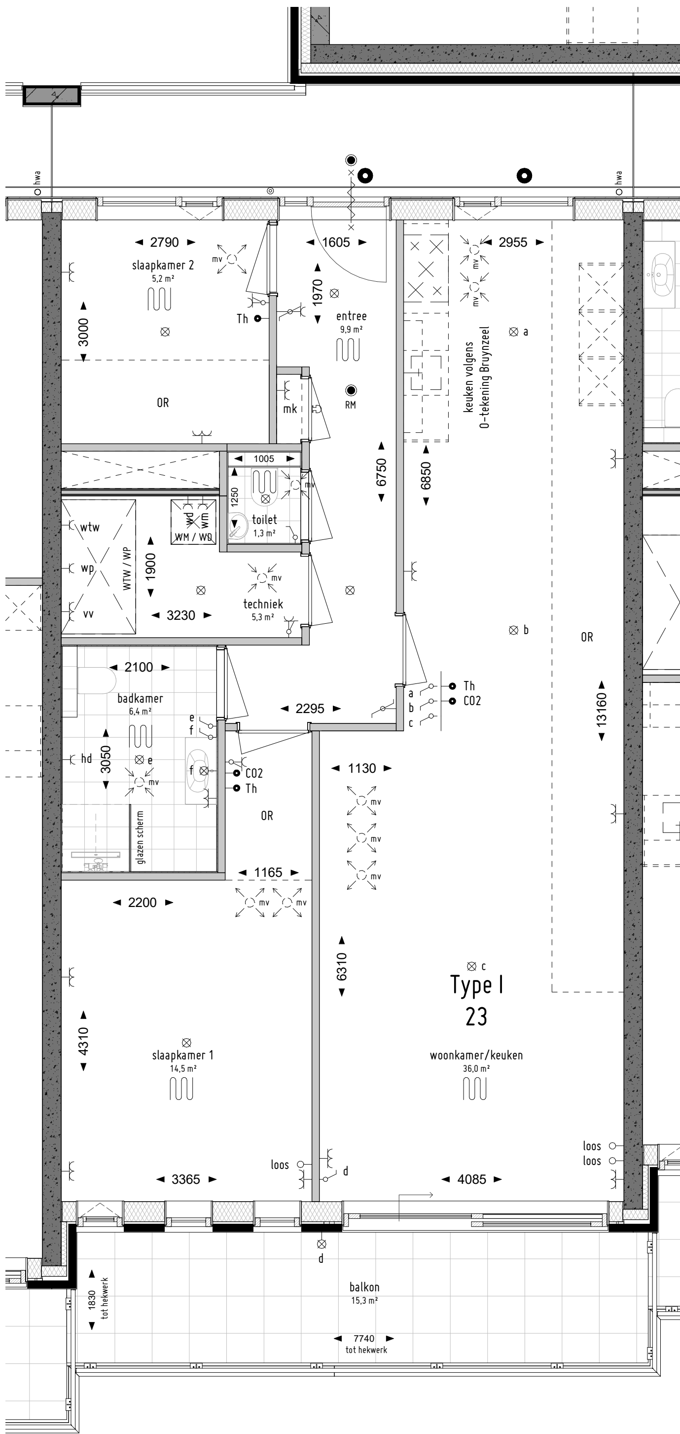
Bouwnummer 23 1 : 50
