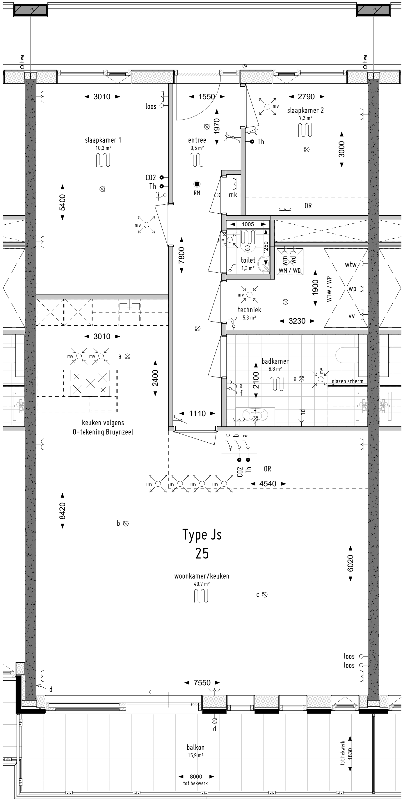
Bouwnummer 25 1 : 50
