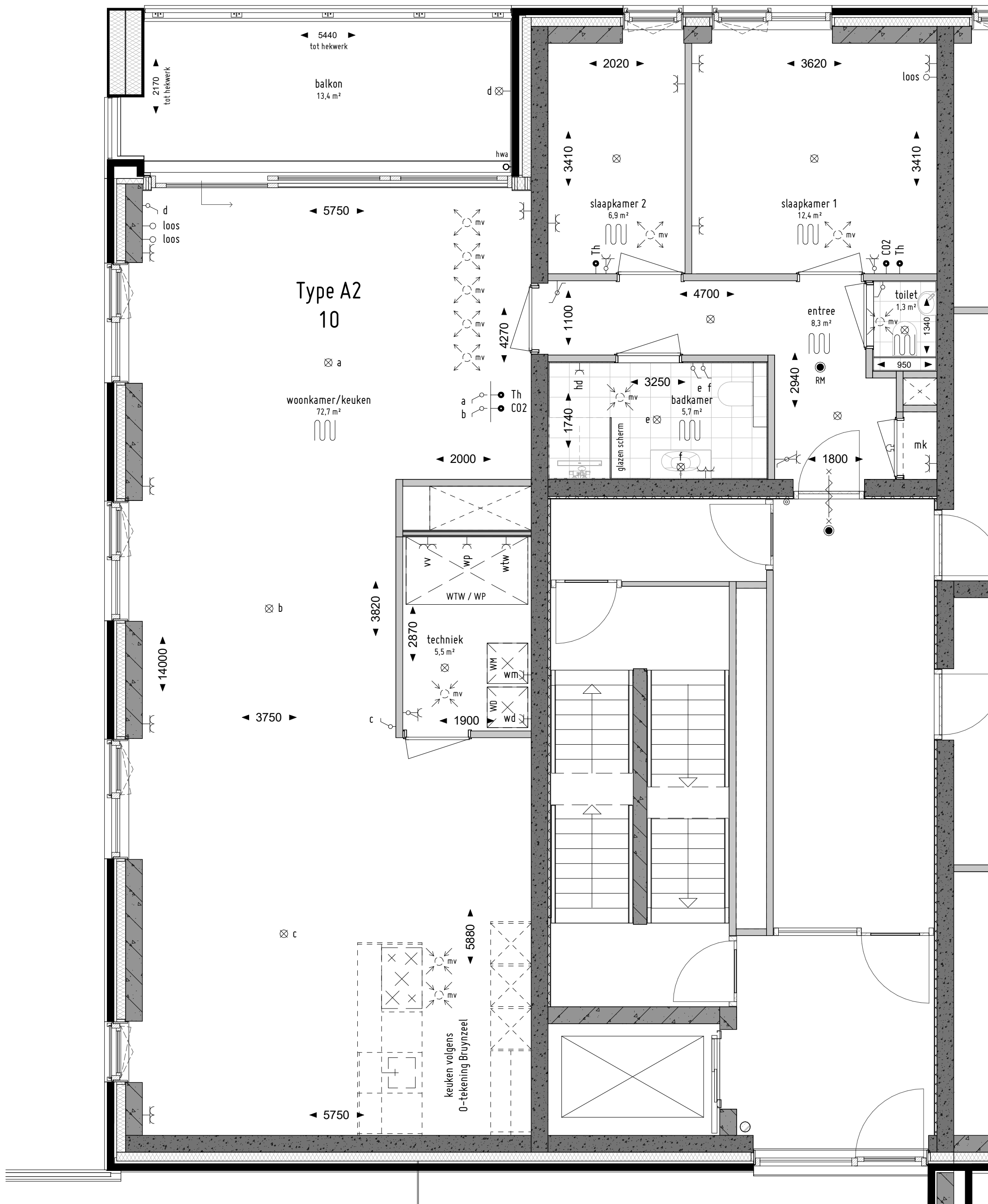
Bouwnummer 10 1 : 50
