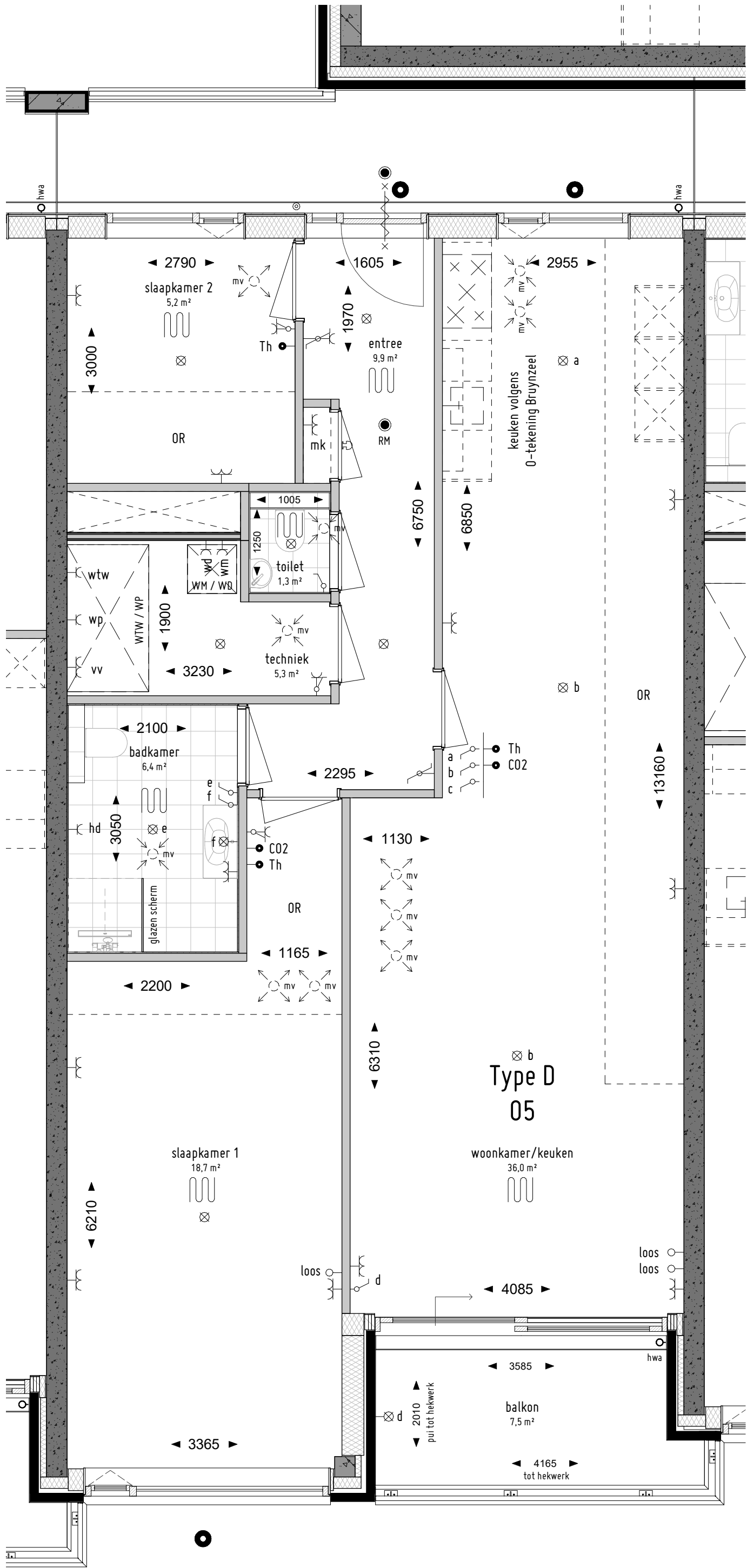
Bouwnummer 05 1 : 50
