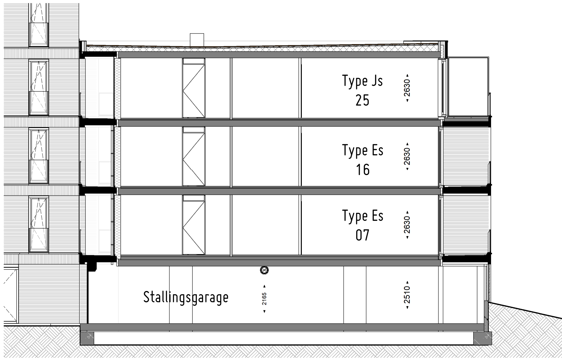
Doorsnede
