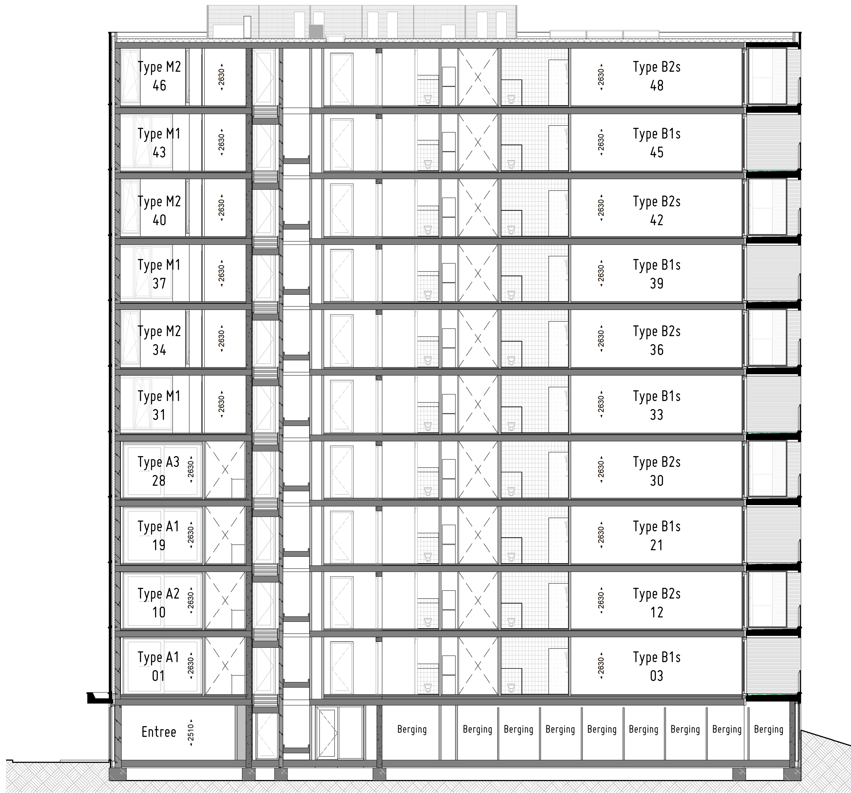
Doorsnede
